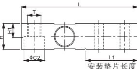
量程 ≤10Klb / 5t: 线缆 φ5.1×6m 量程 ≥15Klb / 10t: 线缆 φ6.1×10m
