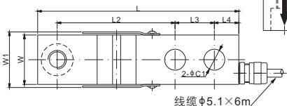
线缆 φ5.1×6m
