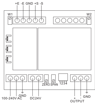
接线图
