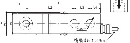
线缆 φ5.1×6m
