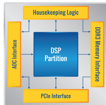
ATS9371 FPGA
