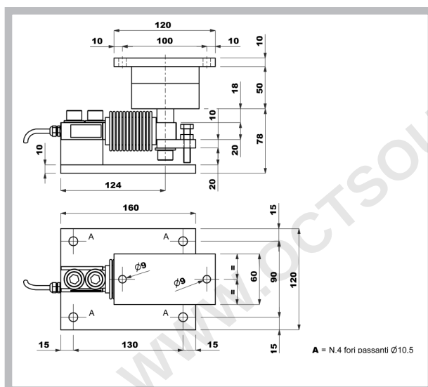
Elastomero per portate 500 - 750 kg
