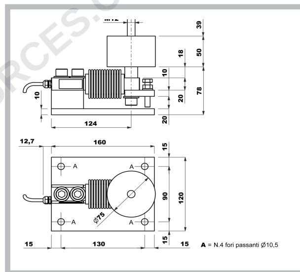
Antivibrante per portate 250 - 300 kg
